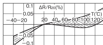
抵抗温度特性 (ゼラニン)
