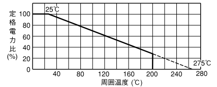
周囲温度と電力軽減曲線
