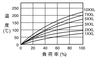
温度上昇例
